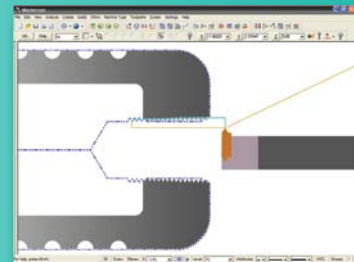
Filetage.
