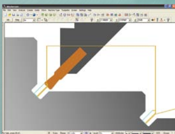
Usinage de gorges sans limite d'orientation.
