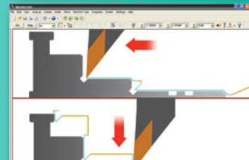
Finition en 2 cycles.
