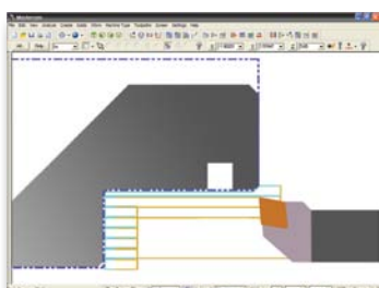
Ebauche d'alésage.
