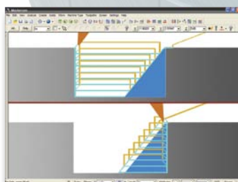
Reconnaissance automatique du brut restant.
