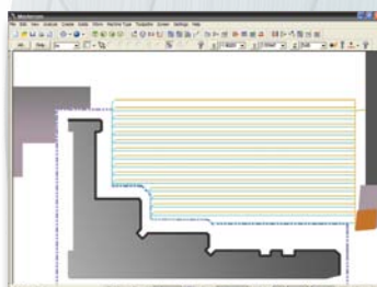
L'outil chariote sans plonger dans les gorges.
